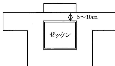
図2 ゼッケンの縫付位置
